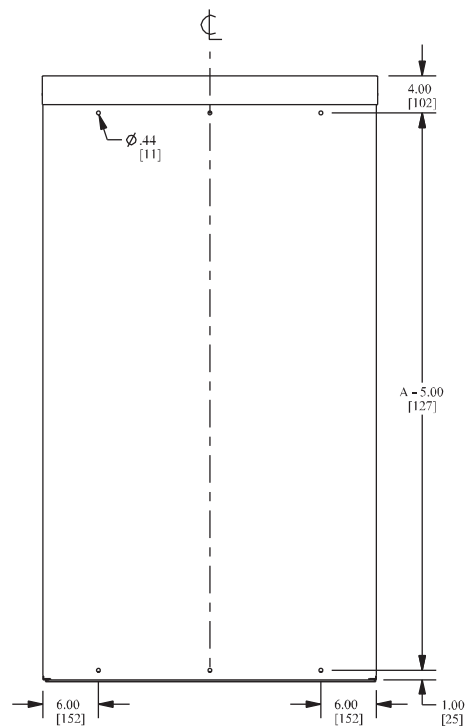
VIEW A-A
